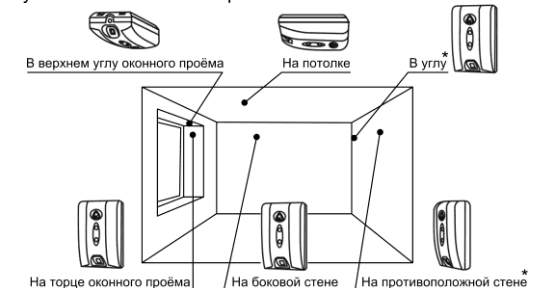
Рис.1 Возможные варианты установки извещателя
