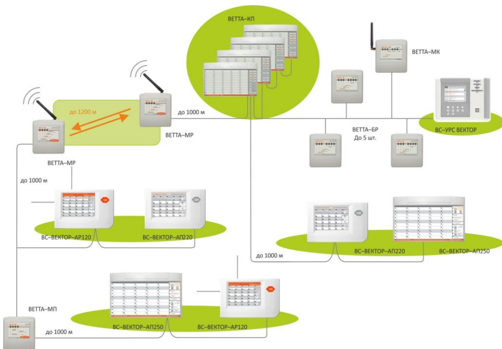
Рис. 2. Пультавая система, система передачи извещений «ВЕТТА – 2020»
